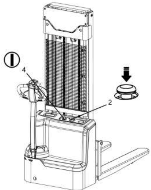
Кнопка подъема/опускания
